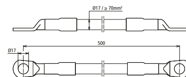
Maßbild D BEB 29-NF / EBS 15-03-17
