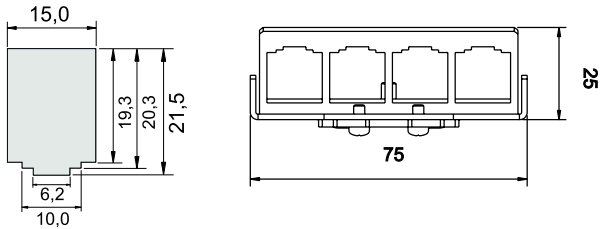
Ausschnittmaße
