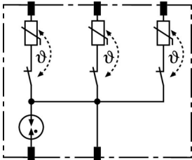
Prinzip Schaltbild DR MOD 4P 255
