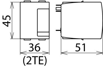
Maßbild DR MOD 4P 255
