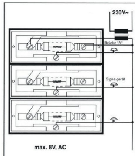
Anschlussplan Circuit diagram Schéma électrique
