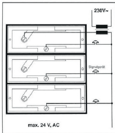
Anschlussplan Circuit diagram Schéma électrique
