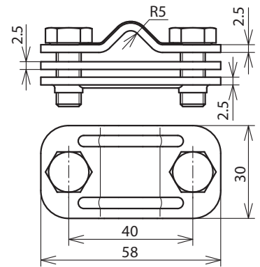
Maßbild UTK 8.10 FL30 ZP V2A
