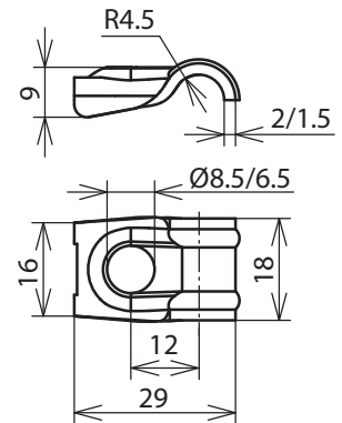
Maßbild UEL DQ 6.10 B8.5 STTZN
