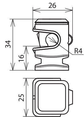
Maßbild LH DS 8 H16 IGM6 BR
