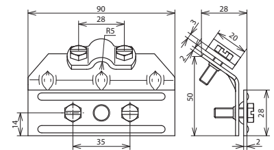
Maßbild SGK ZS 7.10 KB3.13 CU
