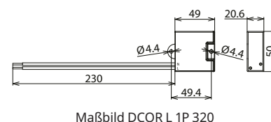
Maßbild DCOR L 1P 320
