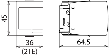
Maßbild DV MOD TT 2P 255
