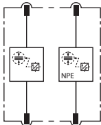
Principalschaltbild DV MOD TT 2P 255
