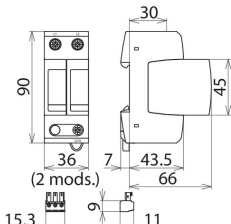
Maßbild DG MU SP 480 3W+G R
