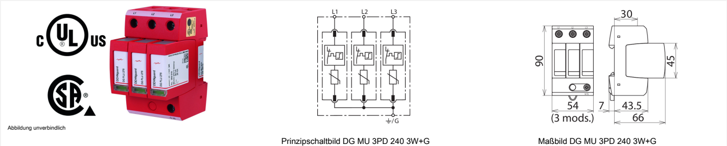
Modularer Überspannungs-Ableiter bestehend aus Basisteil und gesteckten Schutzmodulen für 3 Phase Delta Systeme
