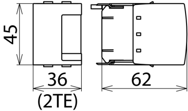
Maßbild DGPH MOD 255
