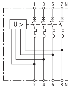
Prinzipschaltbild POP 4 255 C63
