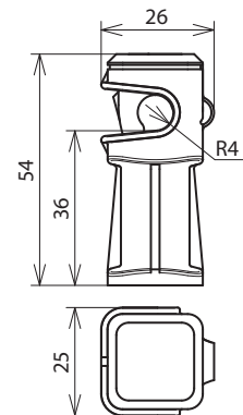
Maßbild LH DS 8 H36 IGM6 GR
