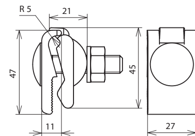
Maßbild AK 4.10 FRM10X45 KBF0.4 12
