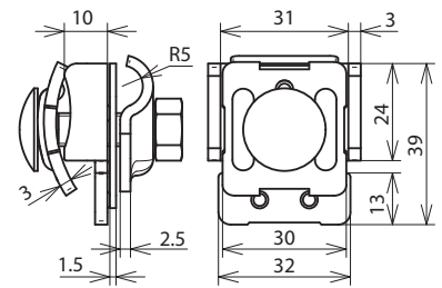
Maßbild ZMFK KB 6.10 KBF0.7 8 STTZN CU
