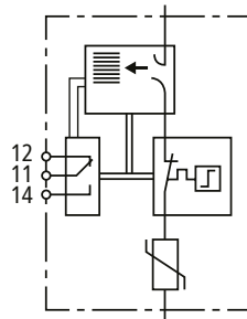
Prinzipschaltbild DG S ACI 275 FM
