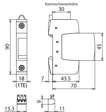
Maßbild DG S ACI 275 FM
