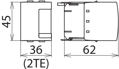
Maßbild DSE MOD PE 60
