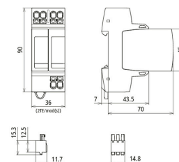
Maßbild DG MP TT 2P ACI 275 FM
