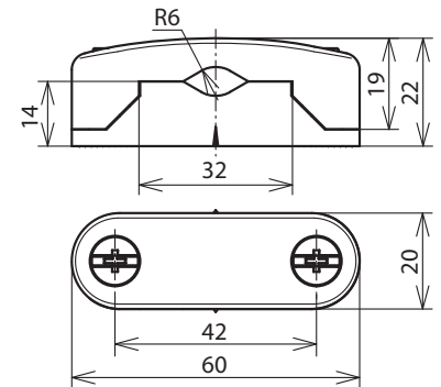
Maßbild LH 6.13 FL30 B10 K GR
