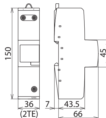
Maßbild DBM 1 440
