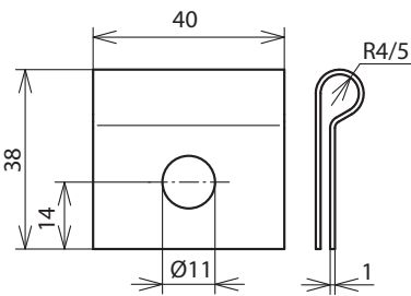
Maßbild KS 10 B11 STTZN
