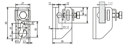
Maßbild FRH 11 6.10 WA11 B7 V2A
