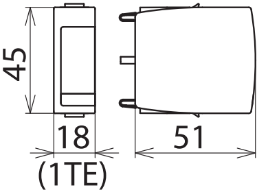
Maßbild DG MOD 440
