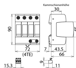
Maßbild DG M H TT 275 FM
