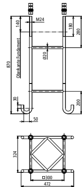
Maßbild AKO TBM FP400
