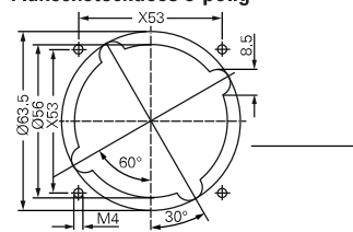
Einbaumaße Flanschsteckdose
