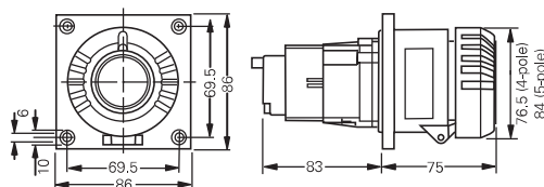
Flanschsteckdose 4/5-polig
