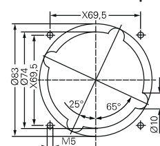
Einbaumaße Flanschsteckdose
