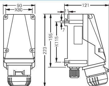
Wandsteckdose 3-polig
