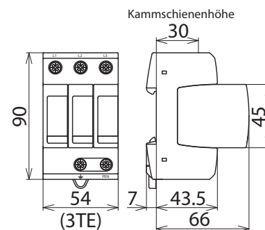
Maßbild DG M WE 600
