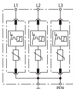
Prinzip Schaltbild DG M WE 600
