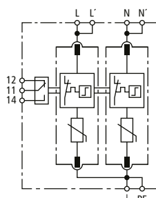
Prinzipschaltbild DG MP TN 150 FM
