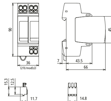
Maßbild DG MP TN 150 FM
