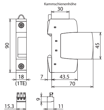
Maßbild DG S ACI 385 FM
