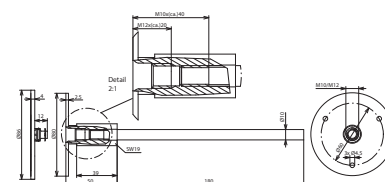
Maßbild EFPM M10 12 V4A L230 V2A
