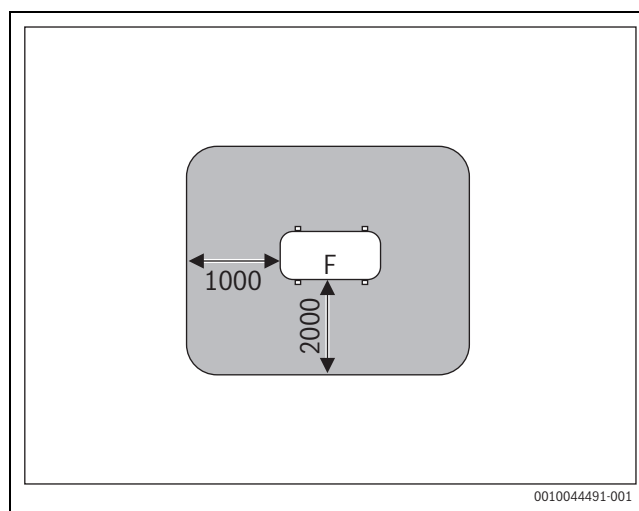
Fig. 2 Volume de protection pour la mise en place au sol sur le terrain ou le toit (dimensions en mm)
