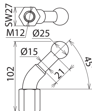
Maßbild KFP 25 W45 M12
