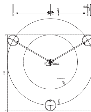
Maßbild DBS KB D40.50 RA1435 STTZN
