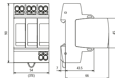
Maßbild DG MP TNC 275
