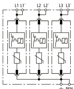
Prinzipschaltbild DG MP TNC 275
