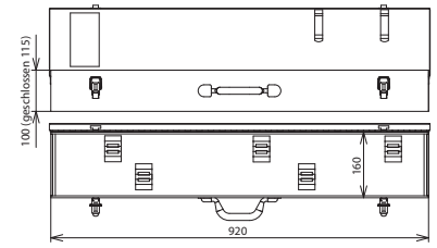
Maßbild SKL 92 16 10
