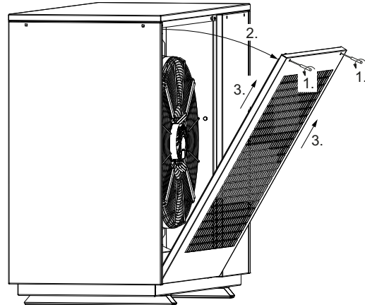
Rys. 7.1: Otwieranie kratownic
