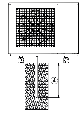
Rys. 6.7: Odpływ kondensatu do podsypki żwirowej
