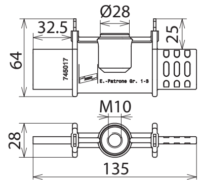
Maßbild EP NH1 3 TI GL M10
