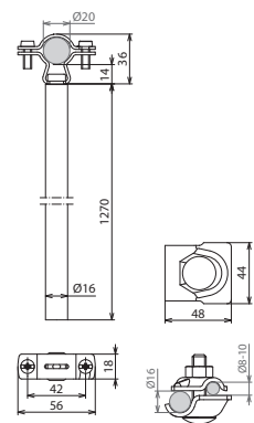
Maßbild DIDH PAE 20 D16 1270 AL V2A
