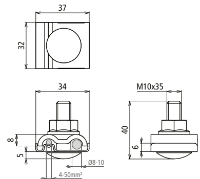
Maßbild KP AQ4 50 DUL 8.10 VKL11 FRSM10
