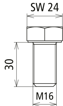
Maßbild D SKS M16X30 V4A
