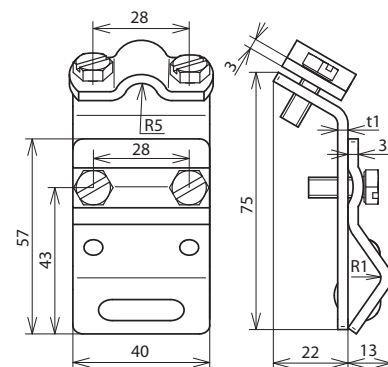
Maßbild DRK ZS 7.10 W13.25 CU
