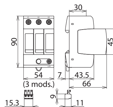
Maßbild DG MU 3PY 480 3W+G R
