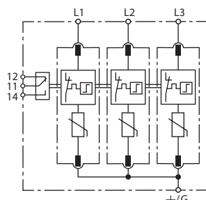
Prinzipschaltbild DG MU 3PY 480 3W+G R
