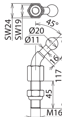
Maßbild KFP 20 W45 M16 45SSM
