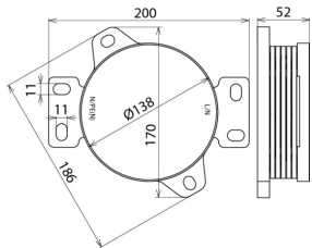
Maßbild DSO 1 255
