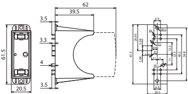
Maßbild DG PCB 275 FM
