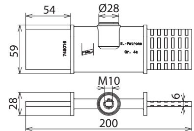
Maßbild EP NH4A TI M10
