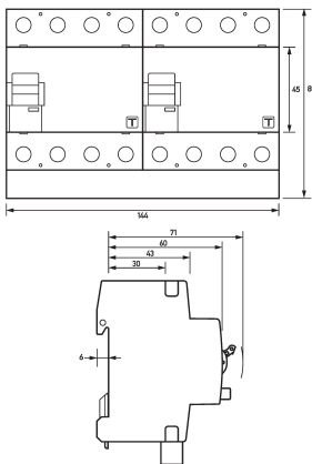
Maßzeichnung Gruppenansicht
