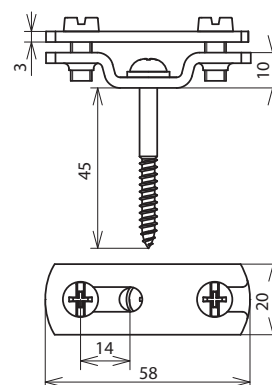
Maßbild FBH ZS 30 B6.5X16 HS5X50 STTZN
